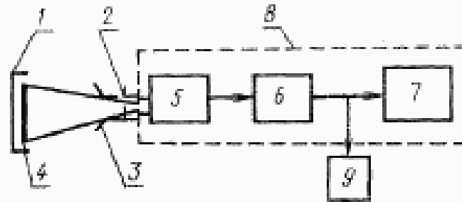
1—световой шкаф; 2—светофильтры; 3—тубус; 4—испытательная таблица; 5—телевизионные камеры; 6—приборы в составе ПТУ; 7—видеоконтрольное устройство; 8—ПТУ; 9—осциллограф
