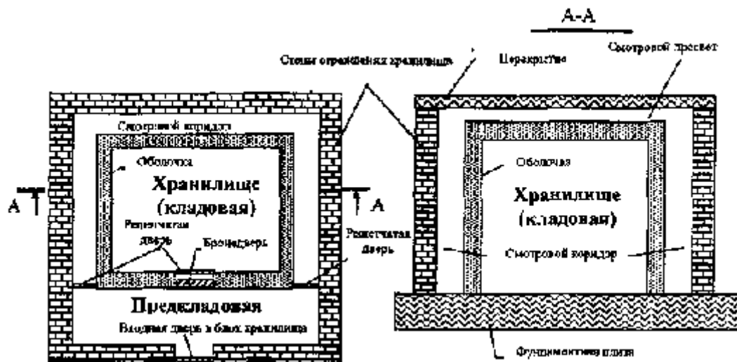
Рисунок П8.1 - Схематическое устройство хранилища ценностей
